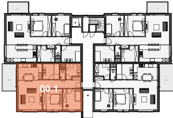
Plan général
